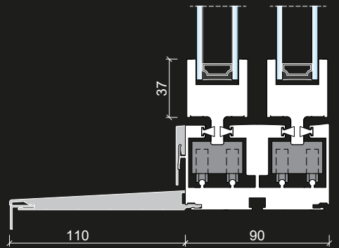
TRAVERSE BASSE AU SOL Avec appui rapporté
