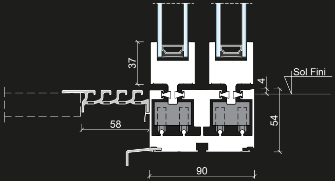
TRAVERSE BASSE AU SOL Avec bavette et caillebotis
