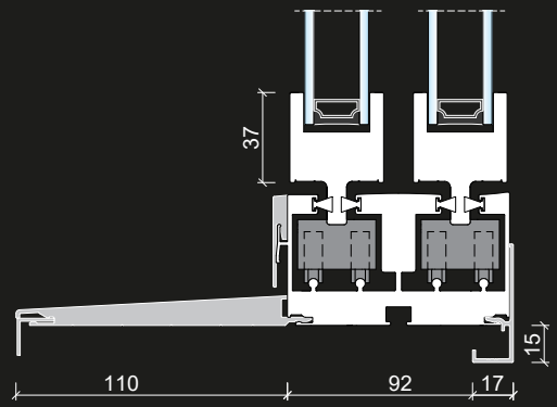
TRAVERSE BASSE SUR ALLÈGE Dormant visible avec appui rapporté
