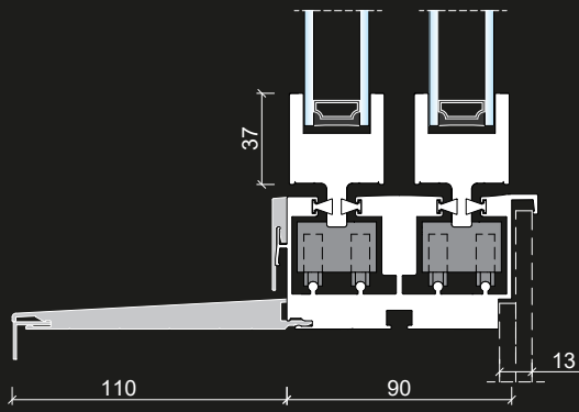
TRAVERSE BASSE SUR ALLÈGE Dormant invisible avec appui rapporté
