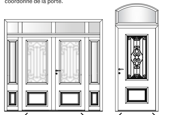
Cormelles-24 Double vantaux avec imposte et fixes en faux ouvrant sans grille.
