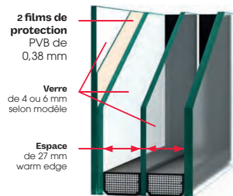
Triple vitrage Disponible en standard uniquement sur certains modèles de la classe P2A et option possible P5A.
