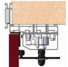
Coupe précadre et capot
