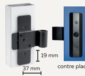
Équerre réglable EASY pour volets à cadre alu uniquement
