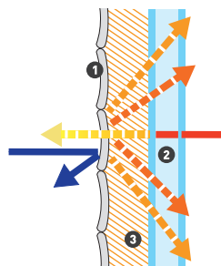
AVEC LAME Thermo-Reflex™
