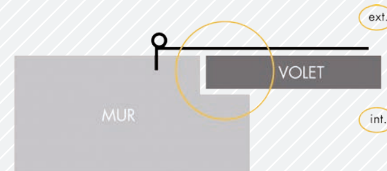
Pose en FEUILLURE Le volet se ferme dans une encoche en haut, à gauche, à droite
