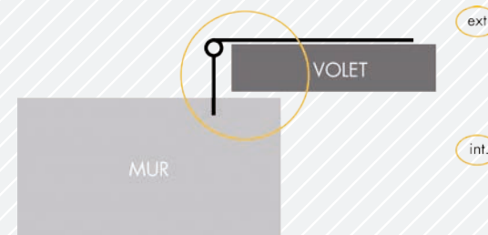
Pose en APPLIQUE Le volet se ferme par-dessus la façade en haut, à gauche, à droite
