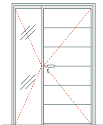
Porte + semi-fixe vitré
