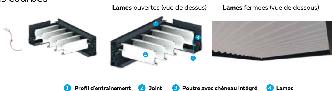
1 Profil d'entraînement 2 Joint 3 Poutre avec chéneau intégré 4 Lames
