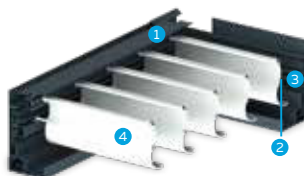
Lames ouvertes (vue de dessus)
