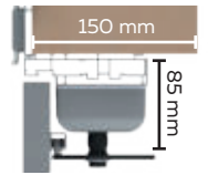
Coupe précadre et capot
