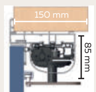
Coupe précadre et capot
