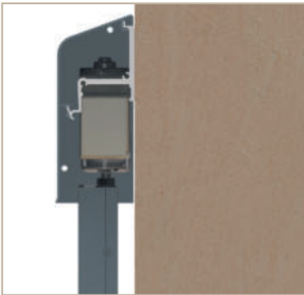
Bandeau (alu laqué ou selon label Qualimarine) allongé pour dissimuler la motorisation
