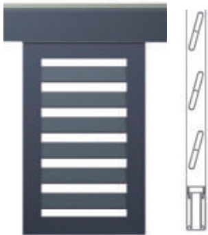
Lames inclinées 68 x 10 mm
