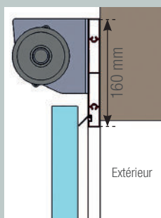
Coupe verticale
