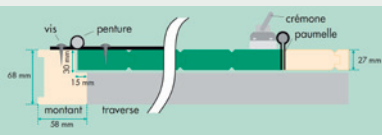
Coupe du bâti Prométhée
