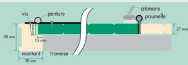
Coupe du bâti Centaure
