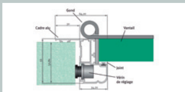
Coupe du bâti rénovation
