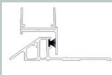
Coupe du seuil et jet d'eau en aluminium
